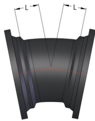
MJ 22-1/2° Bend
