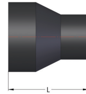
PE x PE Reducer 57M-
